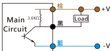
直流3線NPN NO
