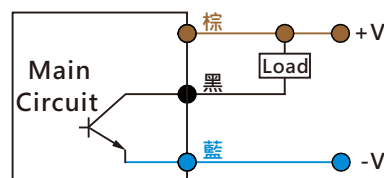
直流3線NPN NO集極開路
